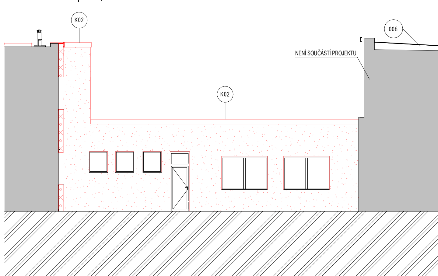
Pohled "Z" - západní, M 1:100
